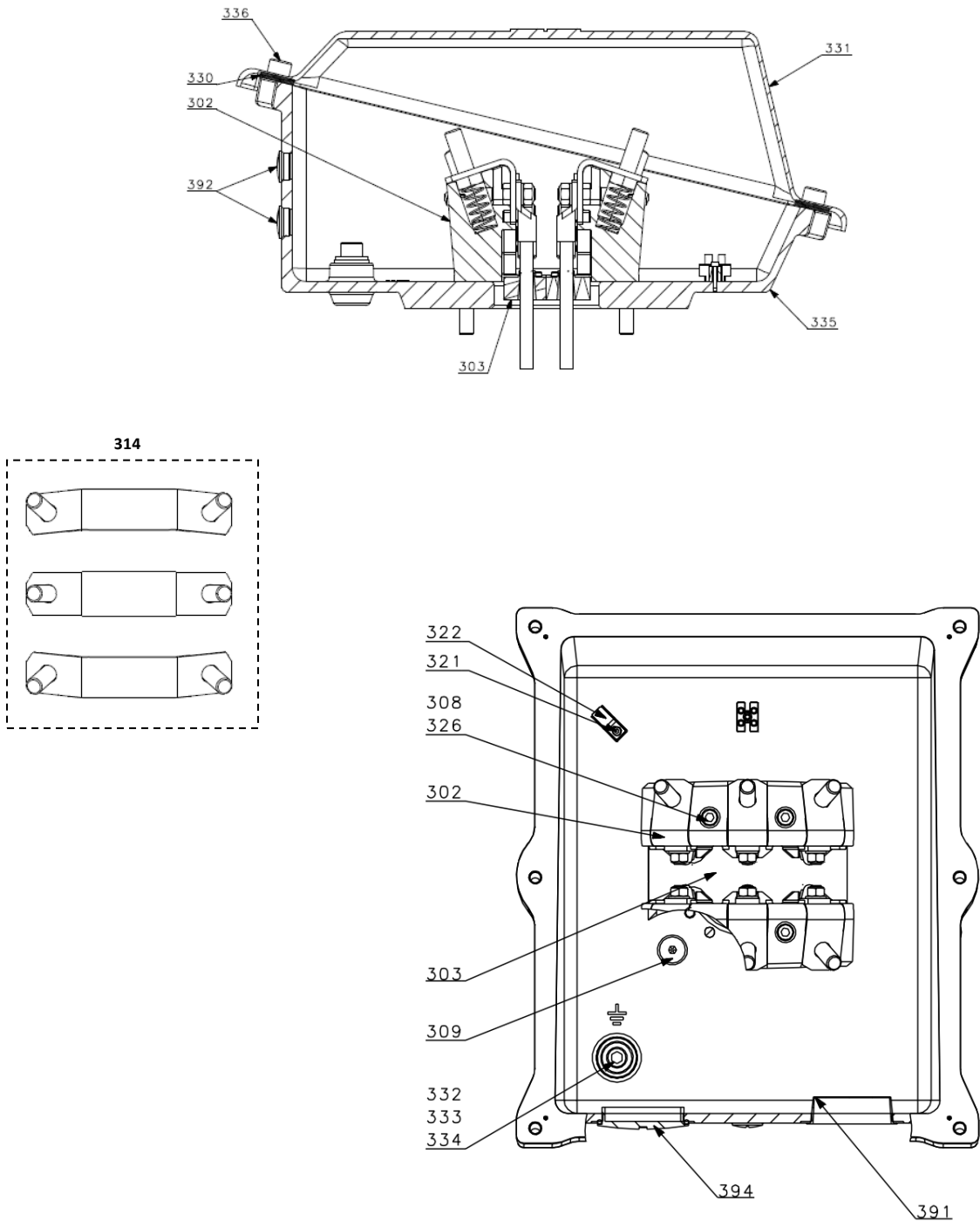
H280-355 (gen. M,MCN) Terminal – 接线终端
